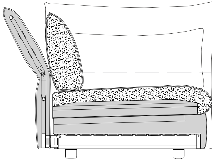
Dwarsdoorsnede samenstelling bekleding
